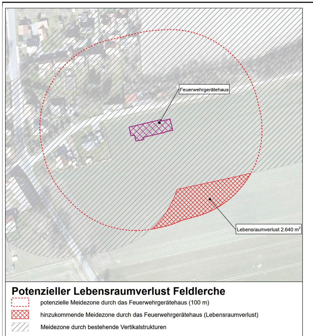
Abb. 2: Konfliktanalyse Feldlerche
